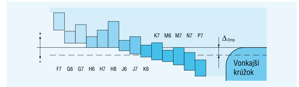
Medzné odchýlky tolerancií priemerov dier
